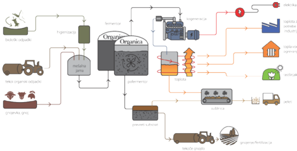
Slika 1: Shematski prikaz nastanka bioplina (Keter Organica d. o. o.)
