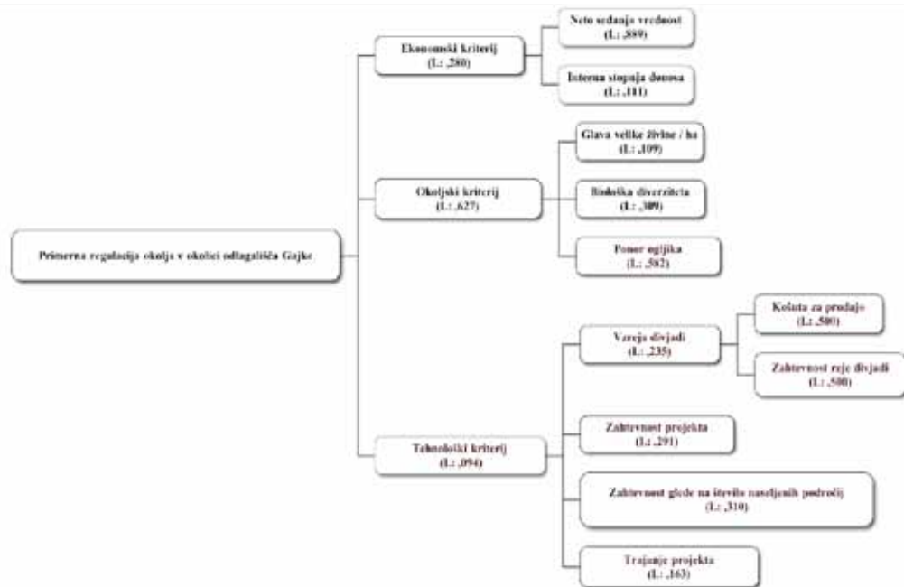
Slika 3.: Hierarhija AHP modela (z izračunanimi prioritetami atributov).
