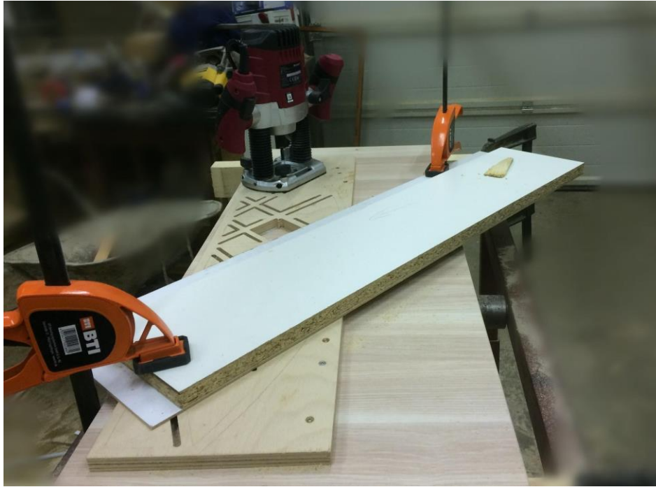
Slika 14: Izrezovanje okvirnega mostu.
