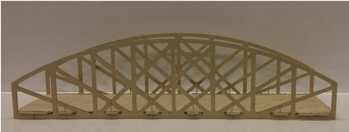
Slika 10: Maketa okvirnega mostu z navpičnimi stebri.
